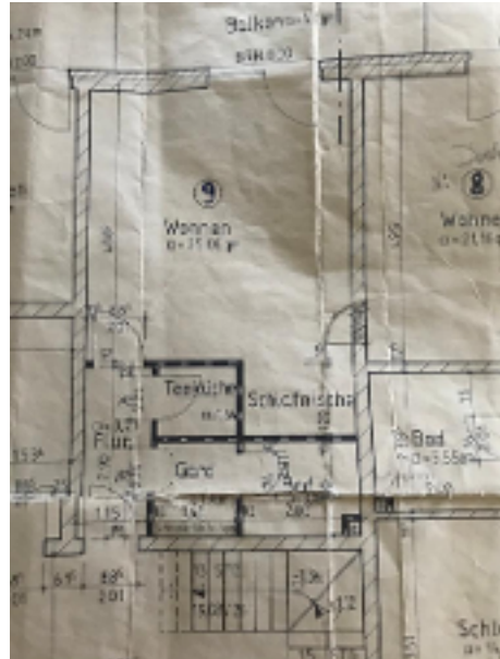
Grundriss
